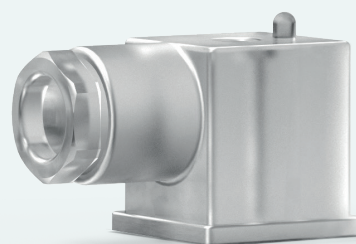
Connettore Led DIN EN 175301-803-A (DIN43650/A) - IP65
